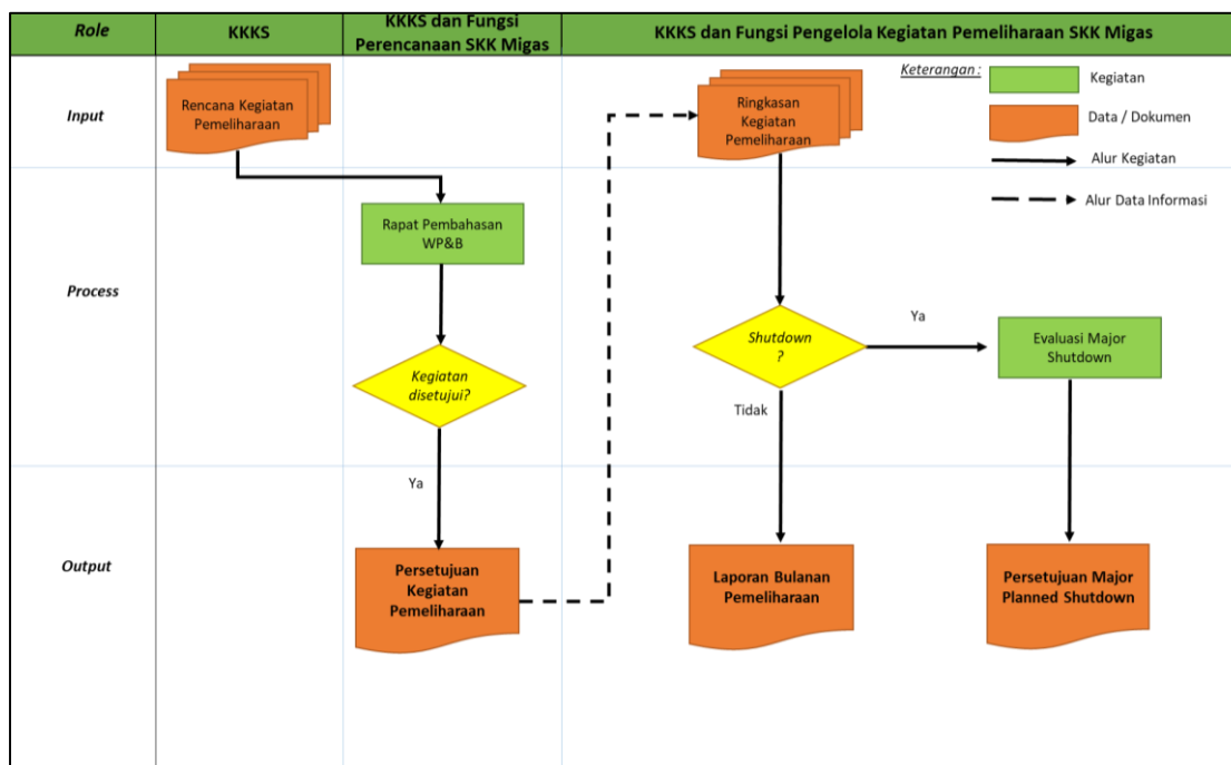
Gambar 3. Perencanaan dan Penjadwalan Kegiatan Pemeliharaan ( Planned Maintenance )
